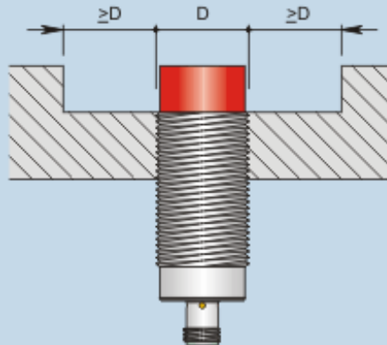
Montaggio sporgente
