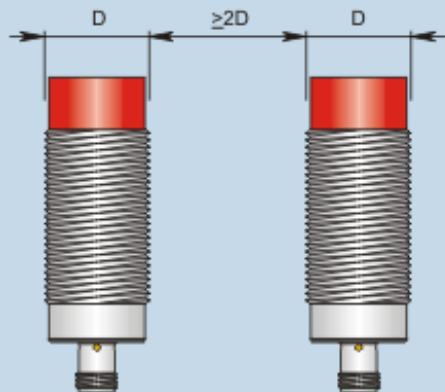
Montaggio affiancato
